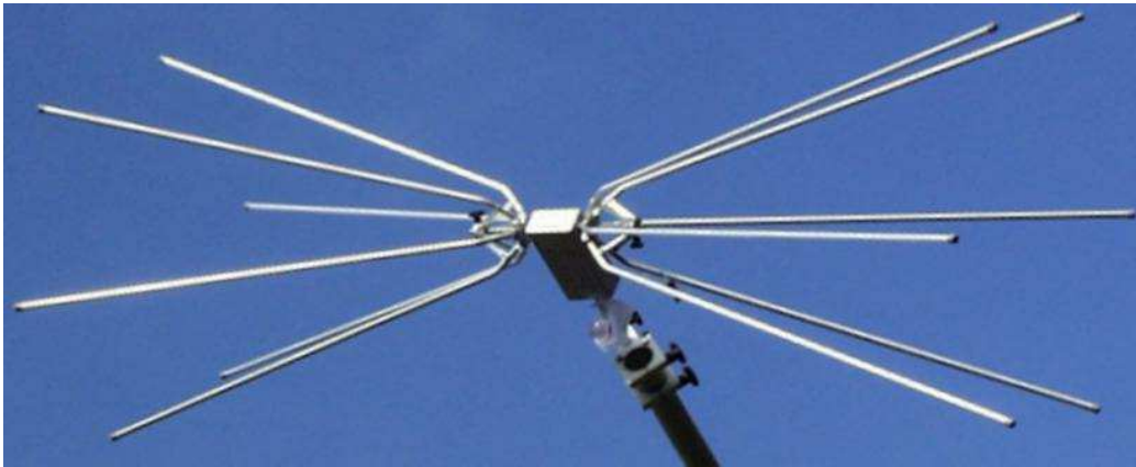
VHBD 9134 Balun mit BBFA 9146 Faltkonus-Elementen (ohne Verlängerungen) VHBD 9134 Balun with BBFA 9146 Collapsible Elements (no extensions mounted)
