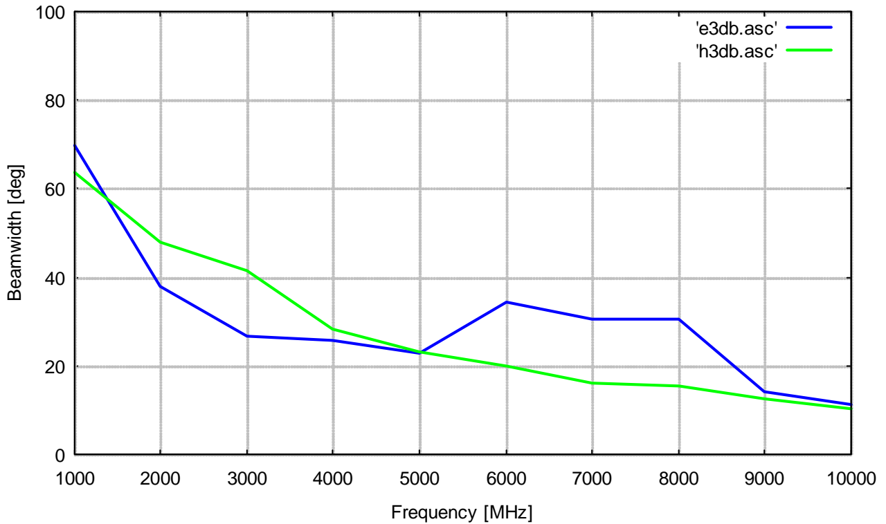
3 dB Beamwidth
