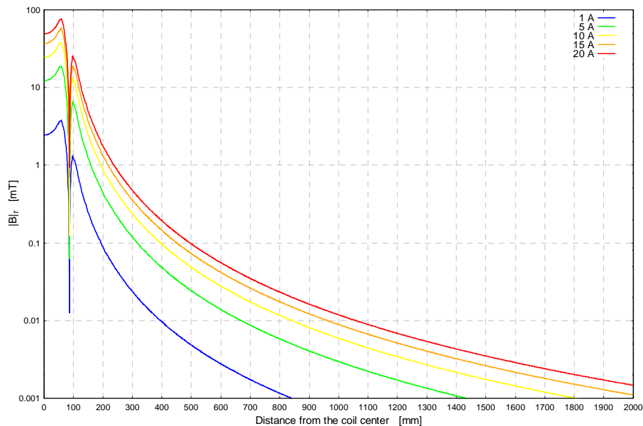
Abb. 4: Der Betrag der magnetischen Flussdichte entlang der r -Achse als Funktion der Entfernung zur Spulenmitte für verschiedenen Stromstärken.
