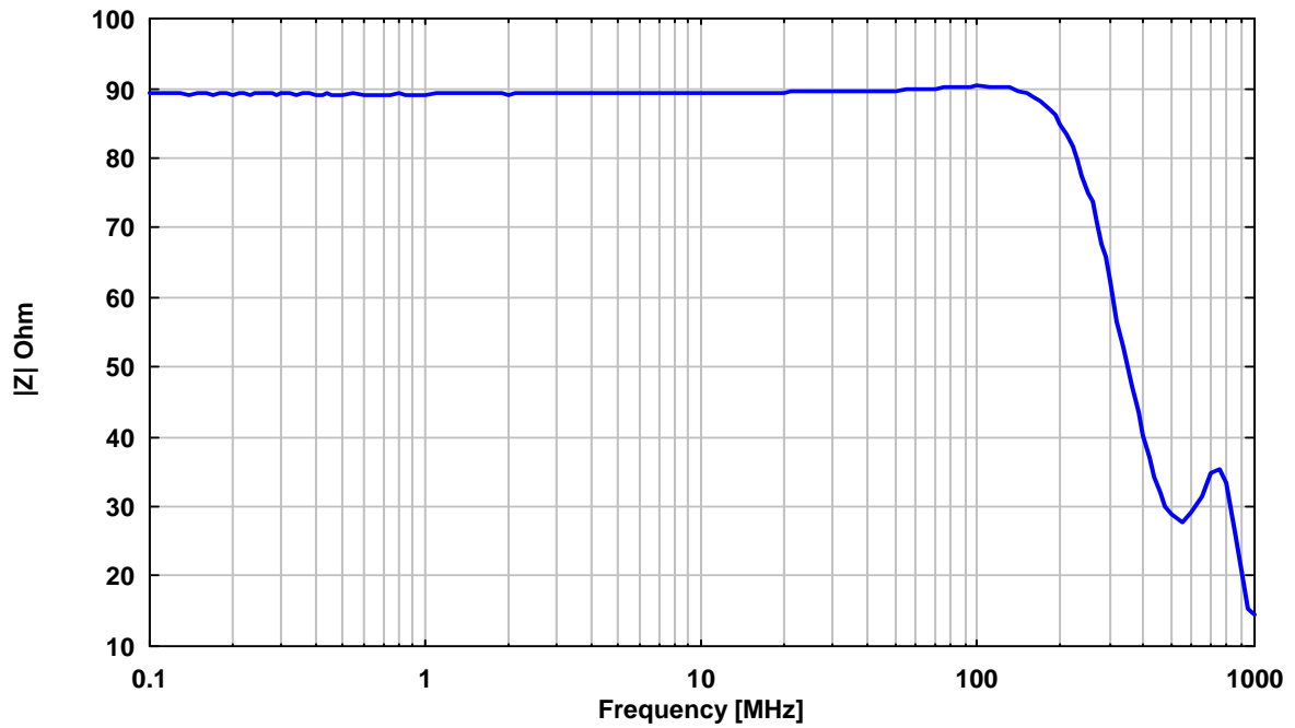
90 Ω Abschlußwiderstand der TEMZ 5232 90 Ohm Termination for TEMZ 5232
