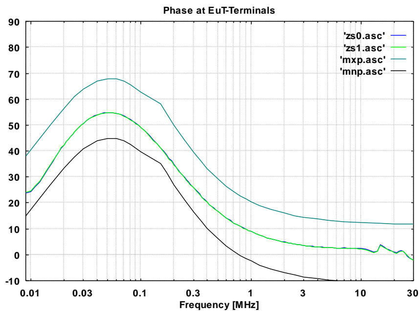
Abb. 8 Phase an den Prüflingsklemmen (SCHUKO), BNC mit 50 Ω Abschluss Phase at the connector for DuT (Schuko), BNC terminated with 50 Ω
