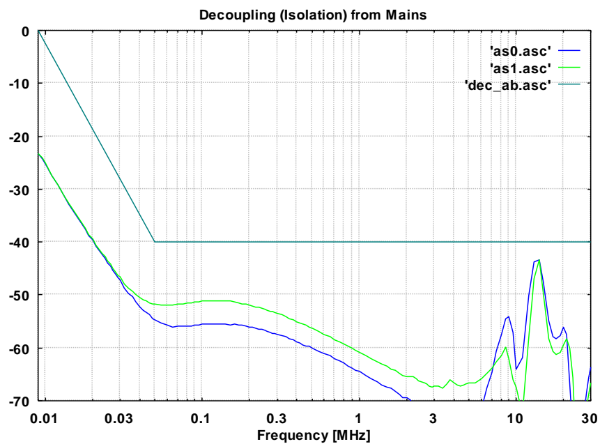
Abb. 10 Entkopplung vom Speisernetz (SCHUKO-Prüflingsklemmen), BNC mit 50 Ω Abschluss/ Decoupling from supply net (Schuko), BNC terminated with 50 Ω
