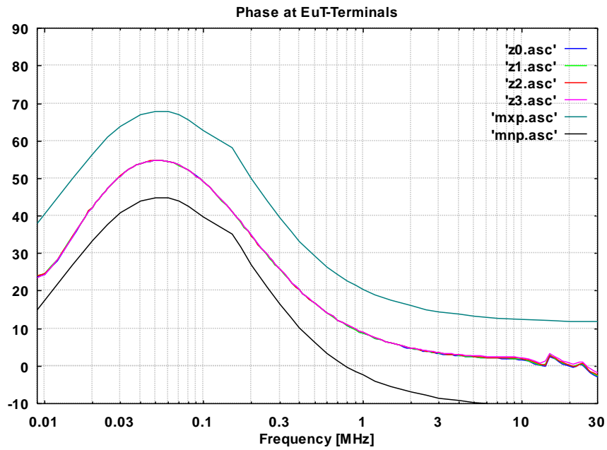
Abb. 5 Phase an den Prüflingsklemmen (CEKON), BNC mit 50 Ω Abschluss Phase at the connector for DuT (CEKON), BNC terminated with 50 Ω
