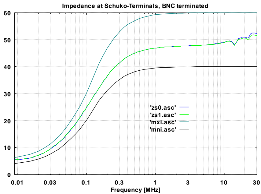
Abb. 7 Impedanz an den Prüflingsklemmen (SCHUKO), BNC mit 50 Ω Abschluss Impedance of connector for DuT (Schuko), BNC terminated with 50 Ω
