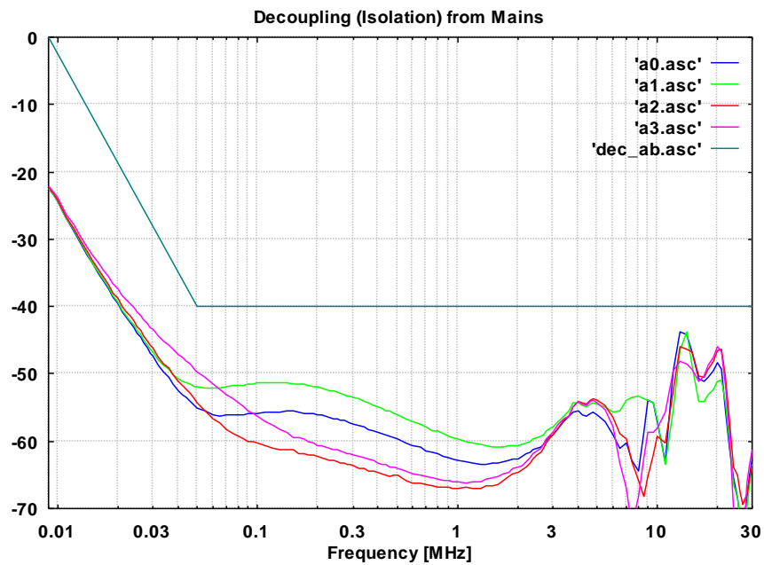
Abb. 9 Entkopplung vom Speisernetz (CEKON-Prüflingsklemmen), BNC mit 50 Ω Abschluss Decoupling from supply net (CEKON), BNC terminated with 50 Ω
