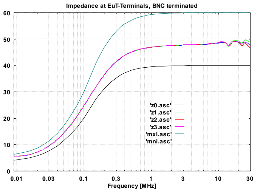
Abb. 4 Impedanz an den Prüflingsklemmen (CEKON), BNC mit 50 Ω Abschluss Impedance of connector for DuT (CEKON), BNC terminated with 50 Ω
