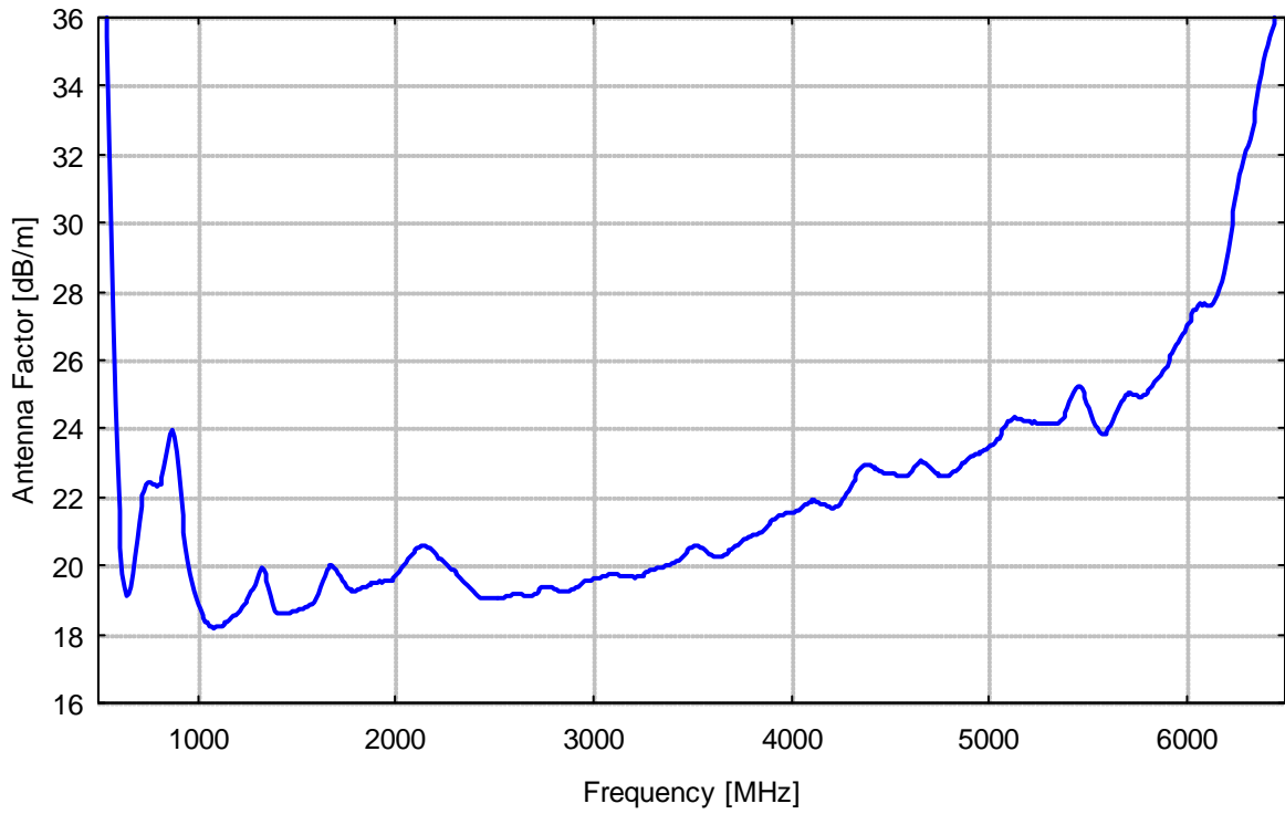
Antennen-Wandlungsmaß
