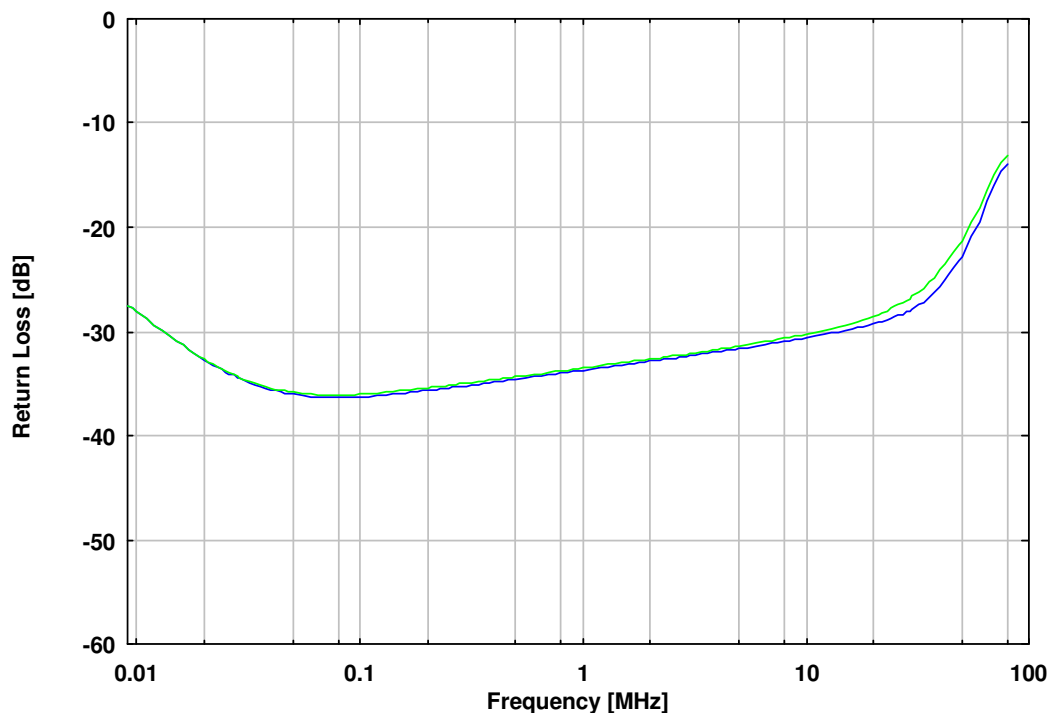
Abb. 2 Anpassung des SY9223-100 (EuT mit 100 \Omega abgeschlossen) Fig. 2: Return loss of SY9223-100 (EuT terminated with 100 \Omega )
