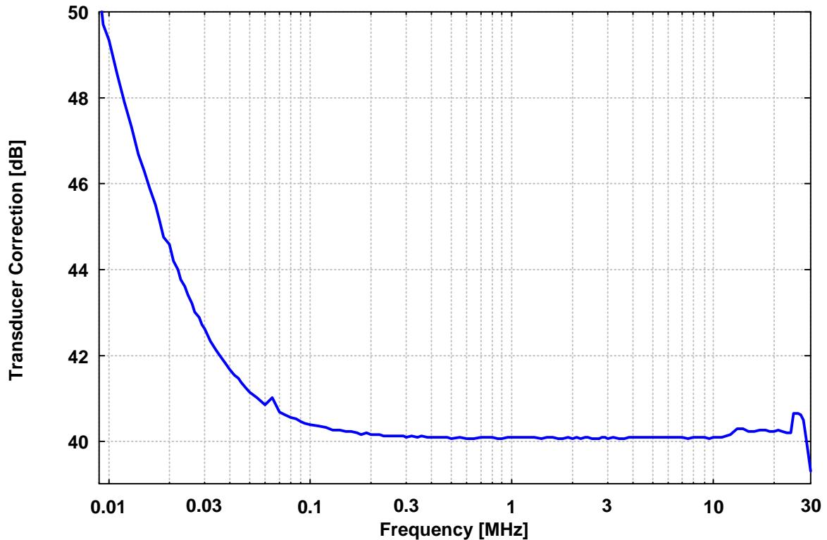
Tastkopf-Wandlungsmaß TK 9422
