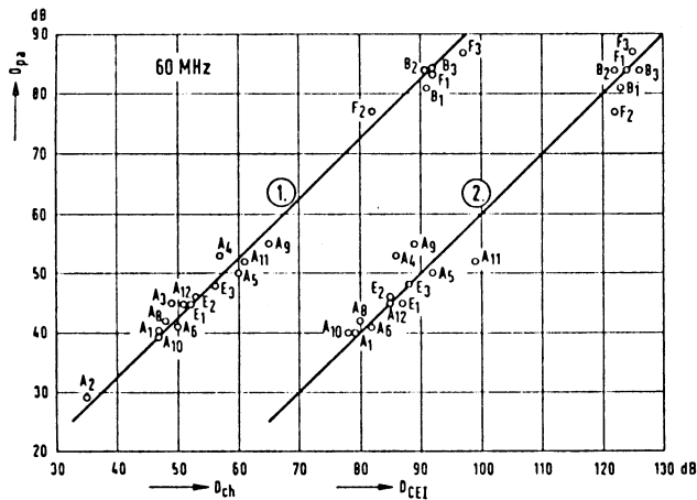
Fig. 9 Efficacité du blindage de câbles coaxiaux à 60 MHz Elektrische Dichtigkeit von Koaxialkabeln bei 60 MHz
