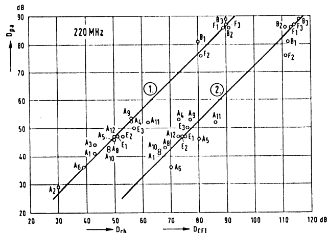
Fig. 11 Efficacité du blindage de câbles coaxiaux à 220 MHz Elektrische Dichtigkeit von Koaxialkabeln bei 220 MHz
