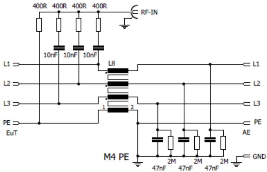
Bild 3: Prinzipschaltbild CDN M4PE 16A 1000V Fig. 3: principal circuitry CDN M4PE 16A 1000V
