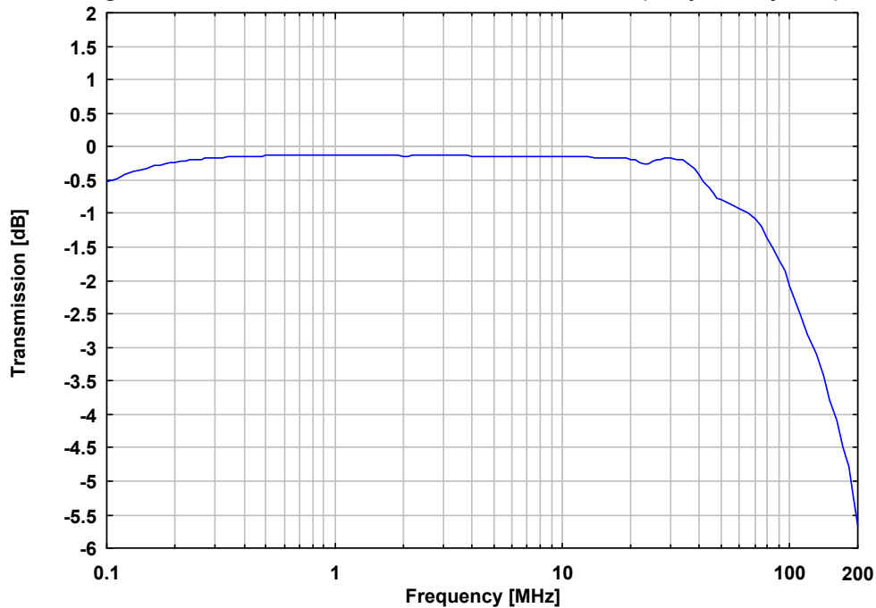
Spannungsteilungsmaß Prüflingsklemmen – N-Buchse (Spezialadapter erforderlich) Voltage division ratio EuT-Terminals to N-connector (adapter required)
